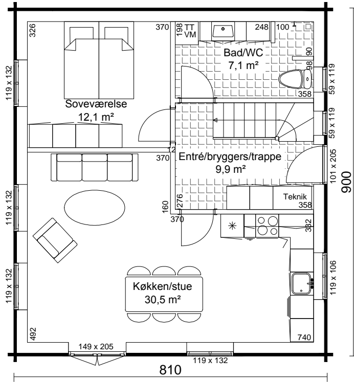
Stueplan
